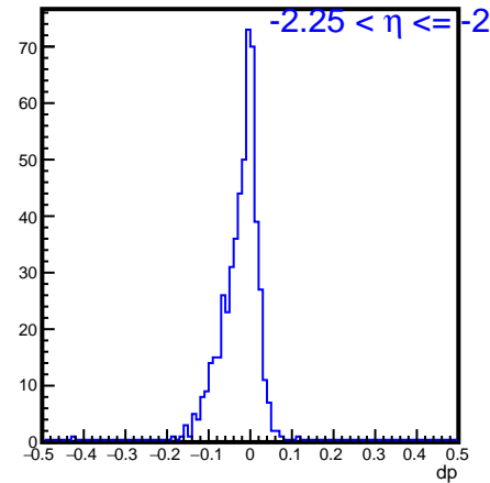
dp_matched_eta_-2.250000_-2.000000
