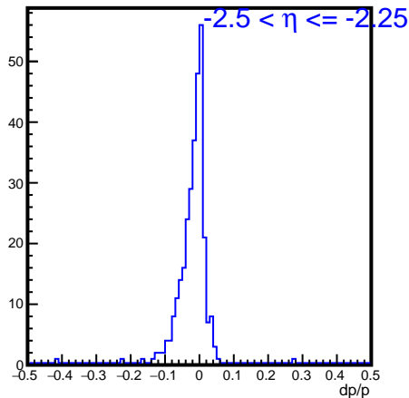
dpoverp_matched_eta_-2.500000_-2.250000
