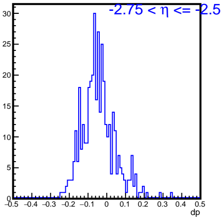
dp_eta_-2.750000_-2.500000
