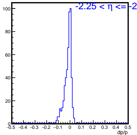
dpoverp_matched_eta_-2.250000_-2.000000
