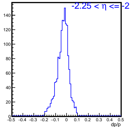
dpoverp_eta_-2.250000_-2.000000
