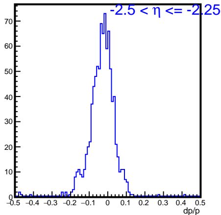
dpoverp_eta_-2.500000_-2.250000
