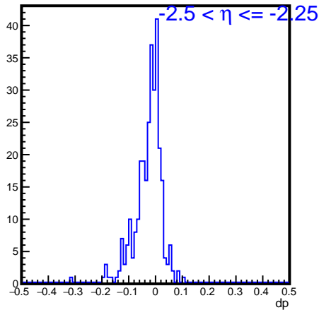
dp_matched_eta_-2.500000_-2.250000
