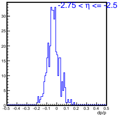
dpoverp_eta_-2.750000_-2.500000
