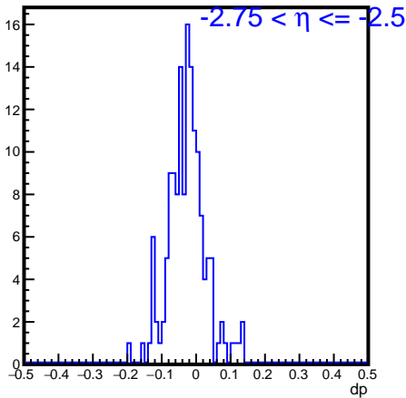
dp_matched_eta_-2.750000_-2.500000
