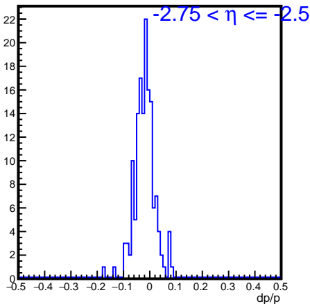
dpoverp_matched_eta_-2.750000_-2.500000
